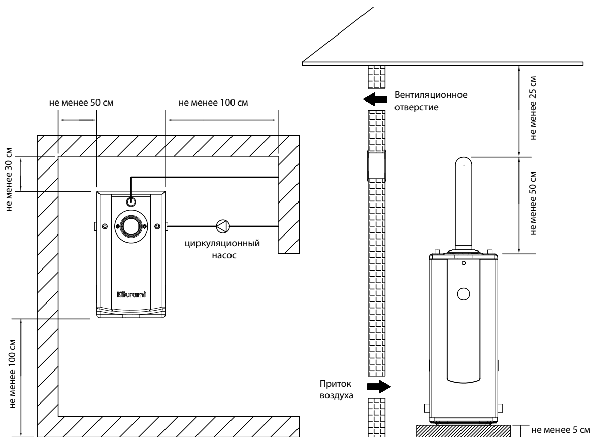
Рисунок 16. Установка котла
