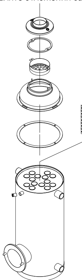
Рисунок 1. Схема доступа к жаротрубным каналам
