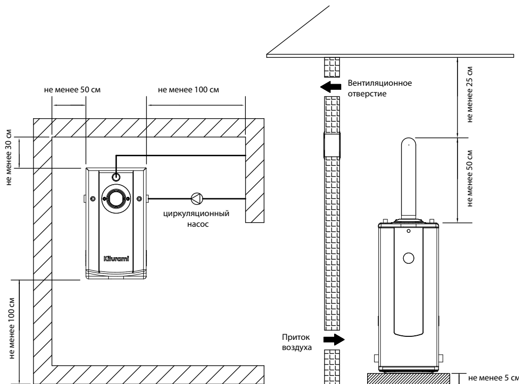
Рисунок 14. Установка котла
