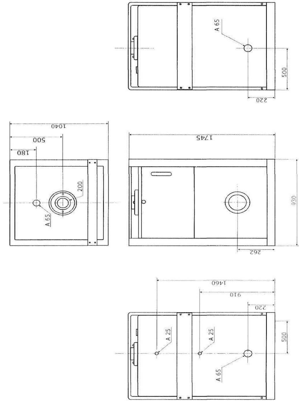
Габаритные и присоединительные размеры котла KSOG-150R с горелкой TGB-150R
